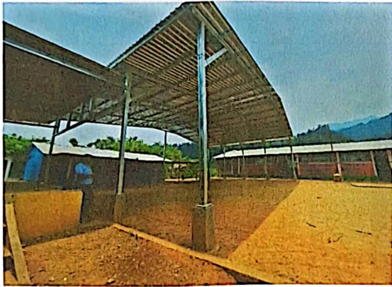
Foto 1: MEJORAMIENTO MODULO 5 (ESCENARIO), CUBIERTA DE LAMINA
