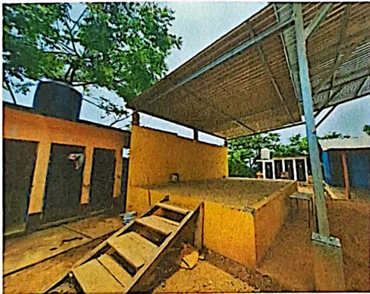
Foto 3: MEJORAMIENTO MODULO 5 (ESCENARIO), ESTRUCTURA DE TECHO
