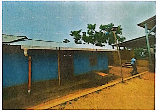
Foto 4: MEJORAMIENTO MODULO 11 Y 5, CANALES Y BAJADAS DE AGUA PLUVIAL
