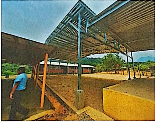
Foto 1: MEJORAMIENTO MODULO 5 (ESCENARIO), ESTRUCTURA DE TECHO
