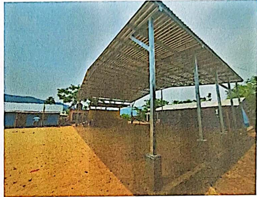
Foto 2: MEJORAMIENTO MODULO 11 (PATIO DEL ESTABLECIMIENTO), LOSA DE PATIO
